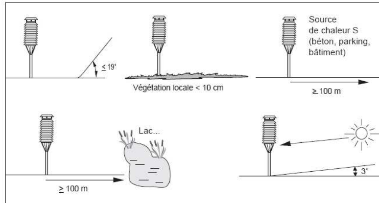
Figure 3 : Critères d'installation d'un abri en classe 1 © Météo-France
